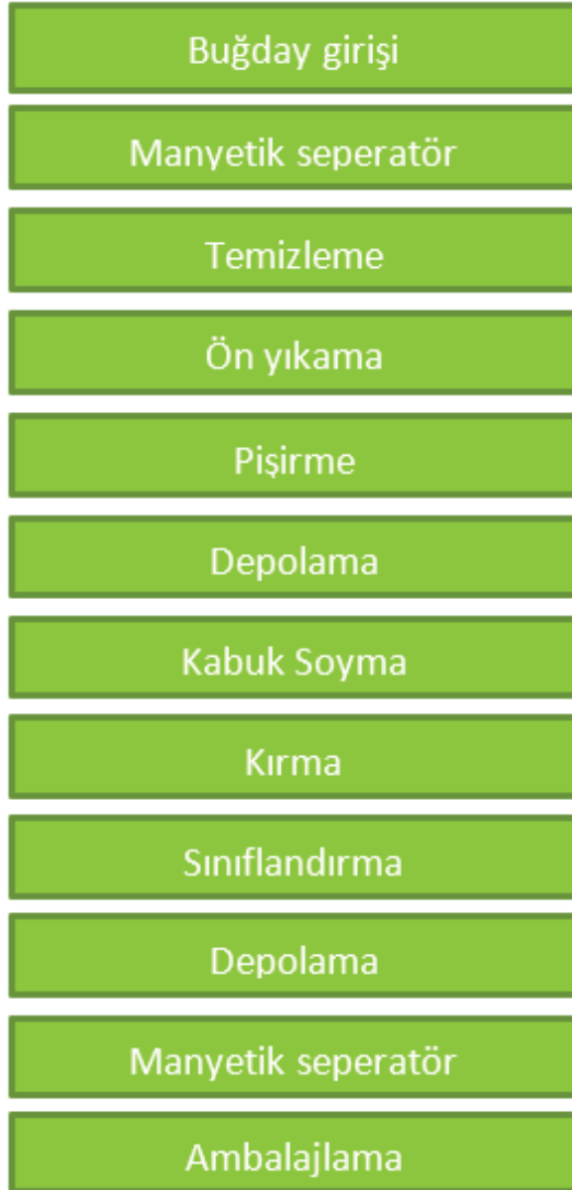
Şekil 1. Bulgur üretim hattı
