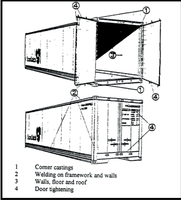
Şekil 4 Görsel Konteyner Kontrolü (Kaynak: IMO MSC/Circ1 787)
