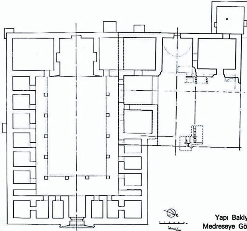
Plan 2: Gökmedrese ve Eski Yapı Kalıntısının Planı (Numan, 1984)
