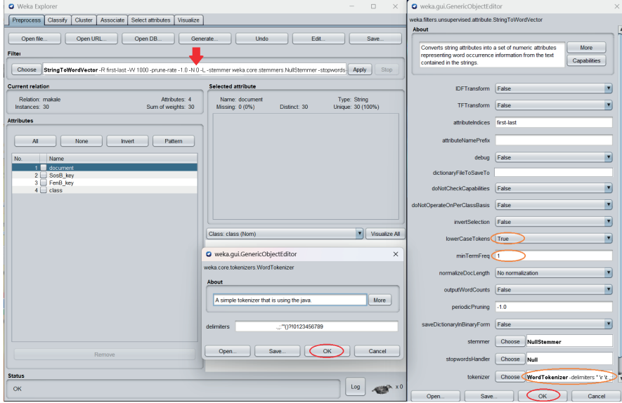
Şekil 7. Veri Ön İşleme Ayarları
