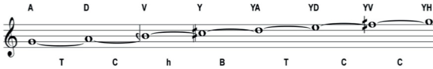
Şekil 6. Şirazi'de Gerdaniye
