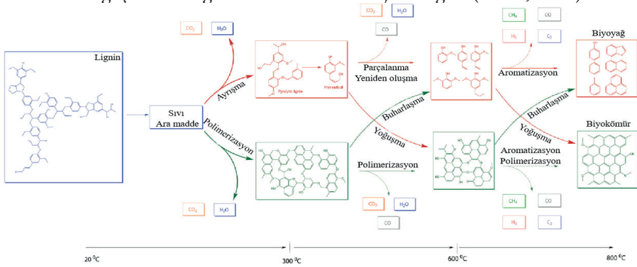
Şekil 5. Ligninin farklı sıcaklıklarda izlediği piroliz adımları (K N vd., 2022)
