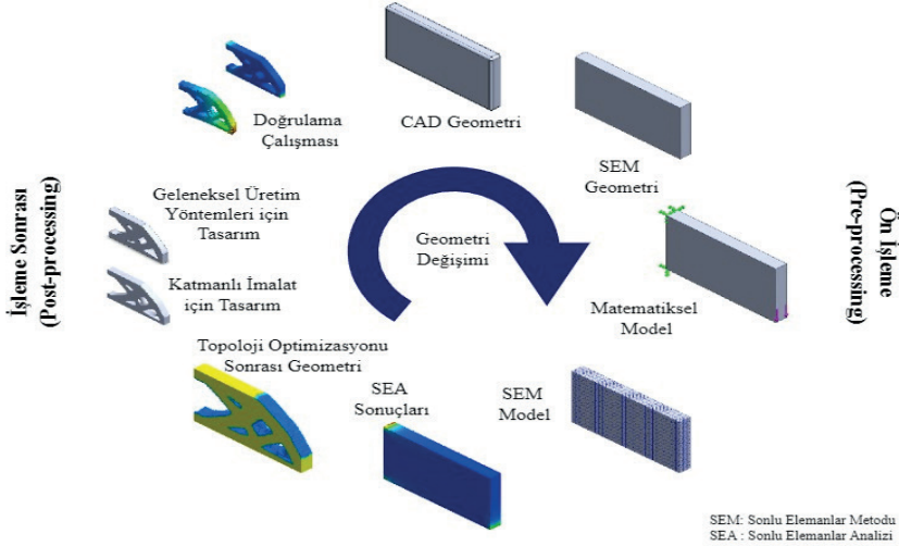
Şekil 3. Topoloji optimizasyonu işlem adımları (Tyflopoulos ve Steinert, 2022)
