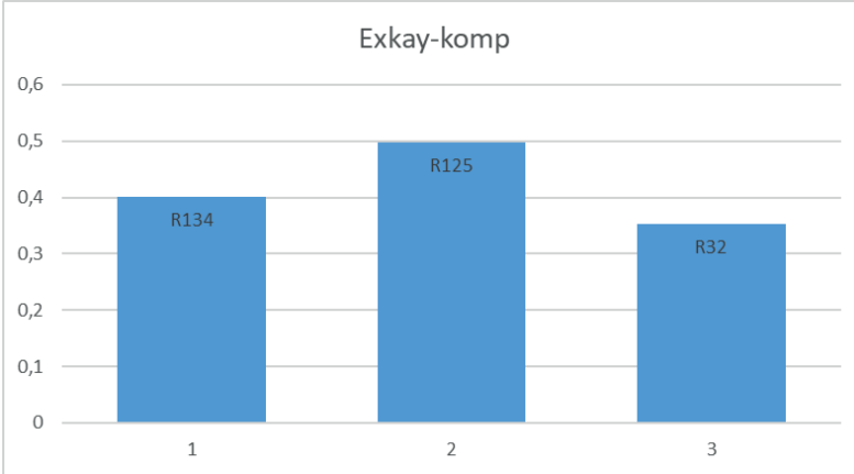
Şekil 9. Isı Pompasının R32, R125 ve R134 için kompresör ekserji kayıpları
