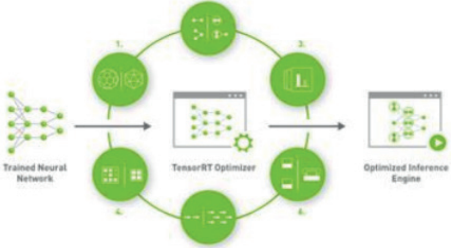
Şekil 16. TensorRT Optimizasyonu
