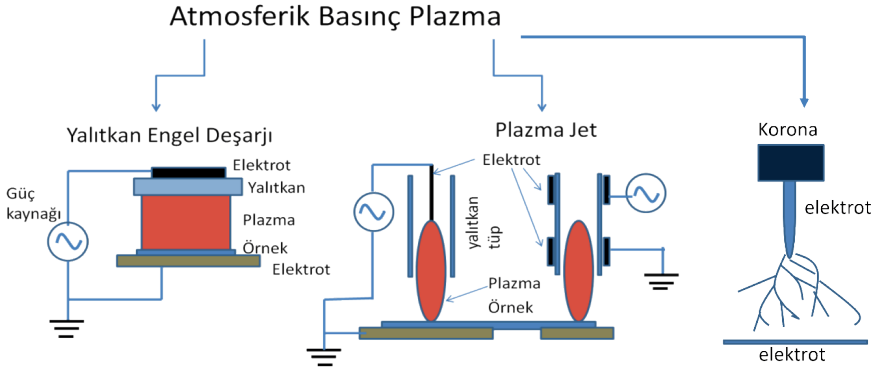
Şekil 2. Atmosferik basınç plazma elde etme yöntemleri
