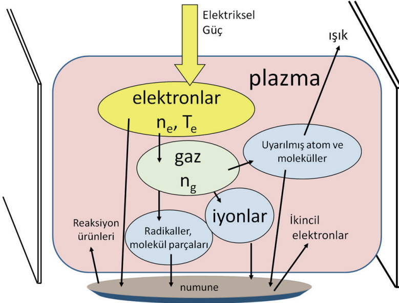
Şekil1. Laboratuvarında plazma (Güleç, 2011).
