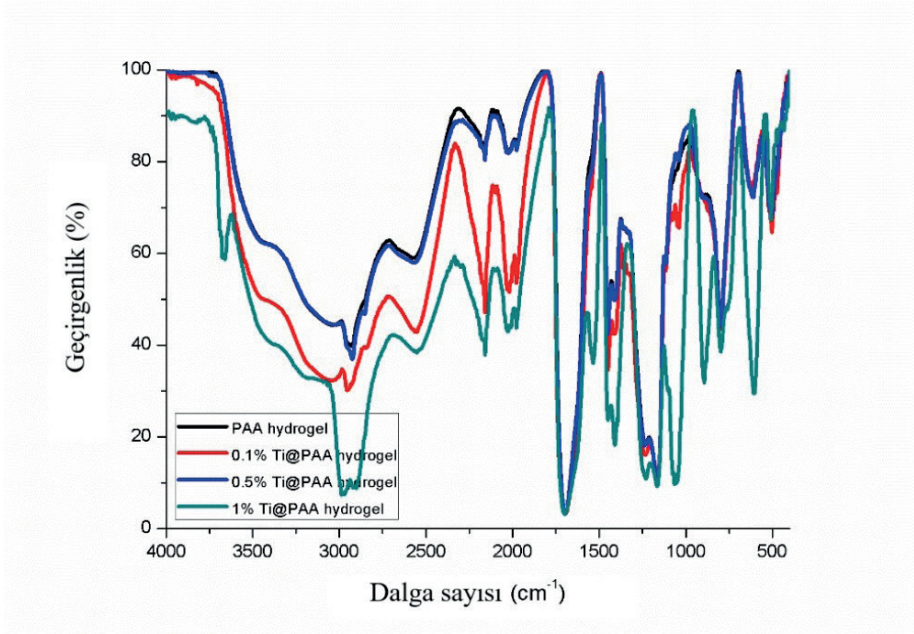
Şekil 5. Katılı ve katkısız PAA hidrojellerine ait FT-IR spektrumları.
