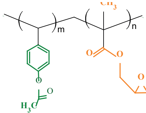
Şekil 1. Poli(Asetoksistiren-ko-glisidilmetakrilat) kopolimerinin kimyasal yapısı
