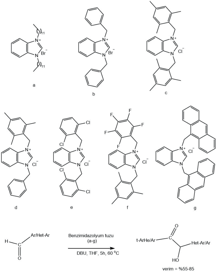
Şekil 4.1. Hacimli benzimidazol tuzlarının aromatik aldehitlerden benzoin sentezine katalitik etkileri
